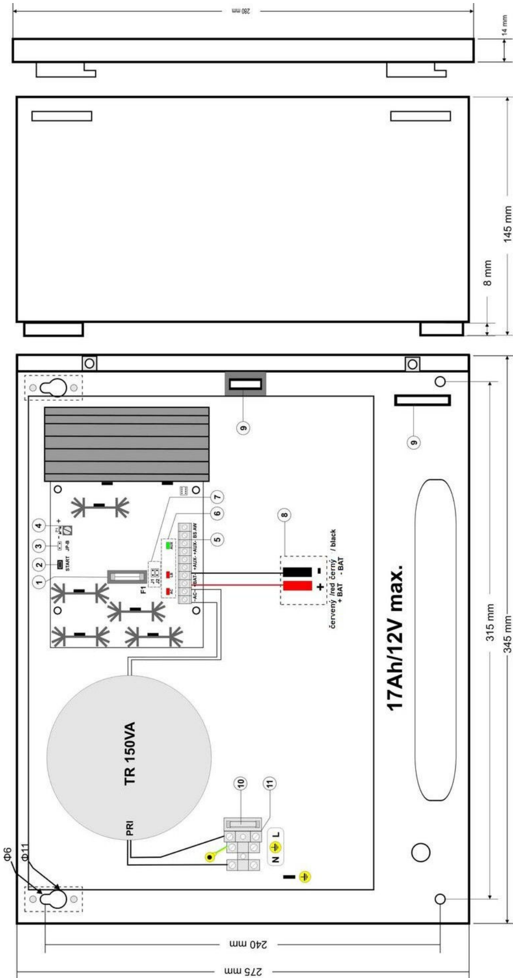
Obr. 2. Pohled na napájecí zdroj.
