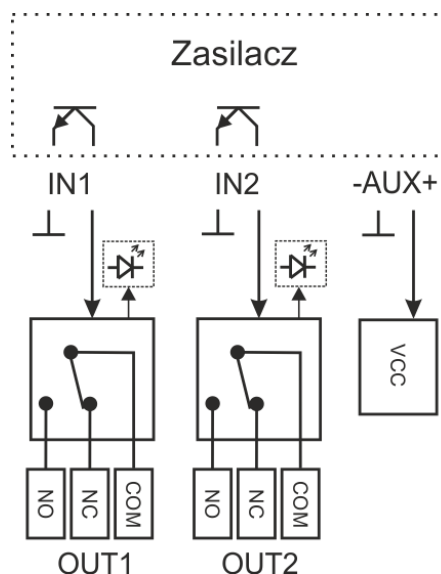
Rys.2. Schemat blokowy.
