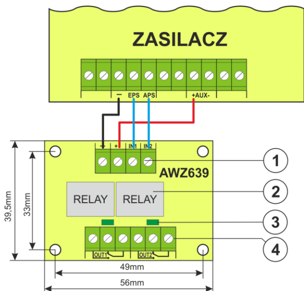
Rys.1. Rysunek modułu.
