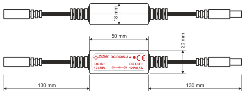
Rys.1. Widok mechaniczny przetwornicy.
