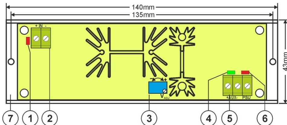
Rys.2. Widok modułu przetwornicy.
