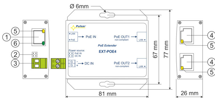
Rys.1. Rysunek urządzenia.
