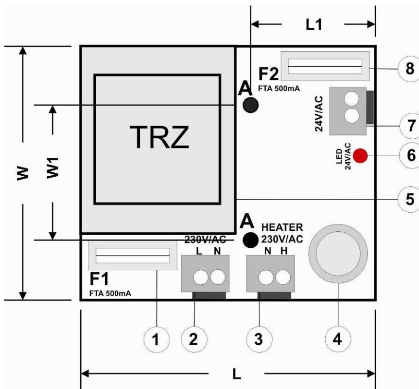
Rys.3. Widok zasilacza.
