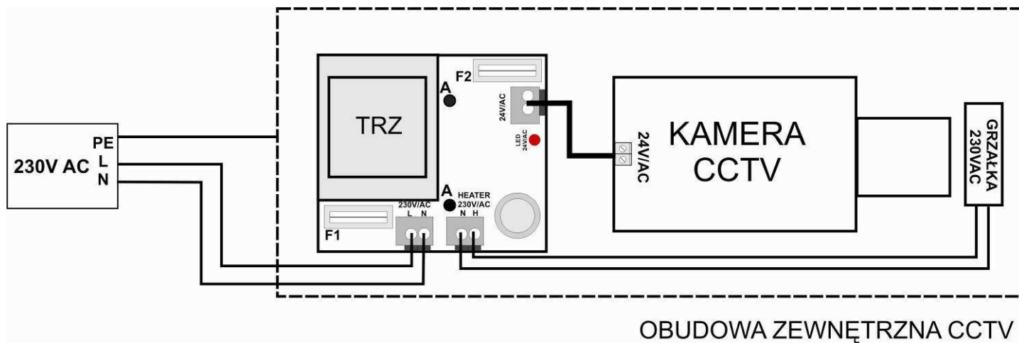
Rys.2. Podłączenie zasilacza: kamera 24V/AC i grzałka 230VAC w obudowie zewnętrznej.
