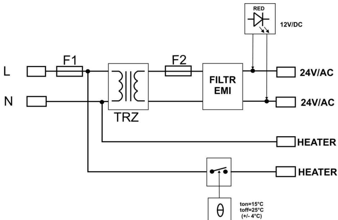
Rys.1. Schemat blokowy zasilacza.
