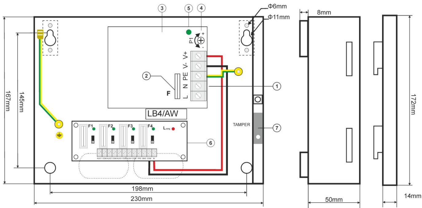
Rys.3. Widok zasilacza.
