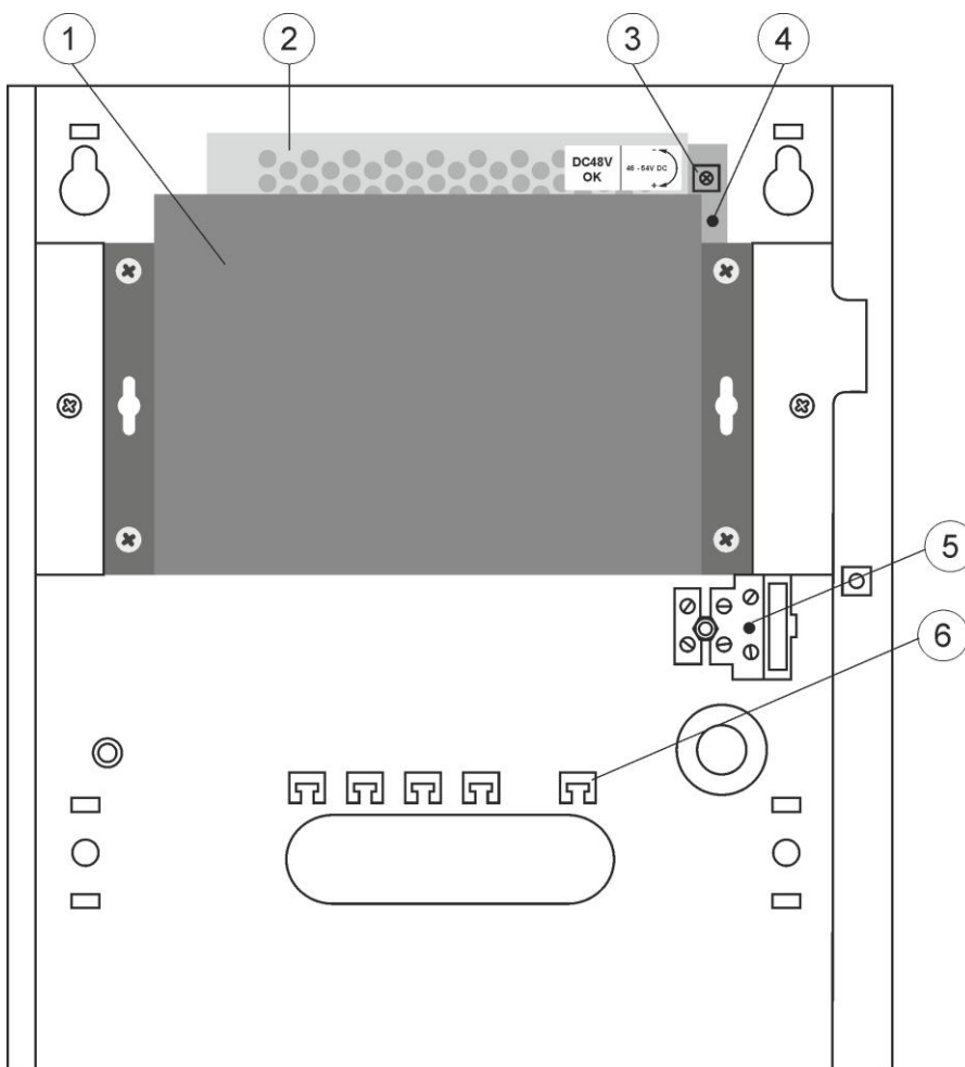
Rys. 2 Widok obudowy.
