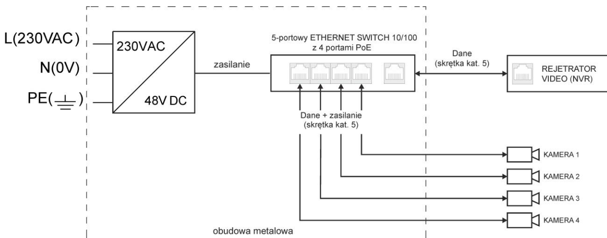
Rys 1. Schemat blokowy.
