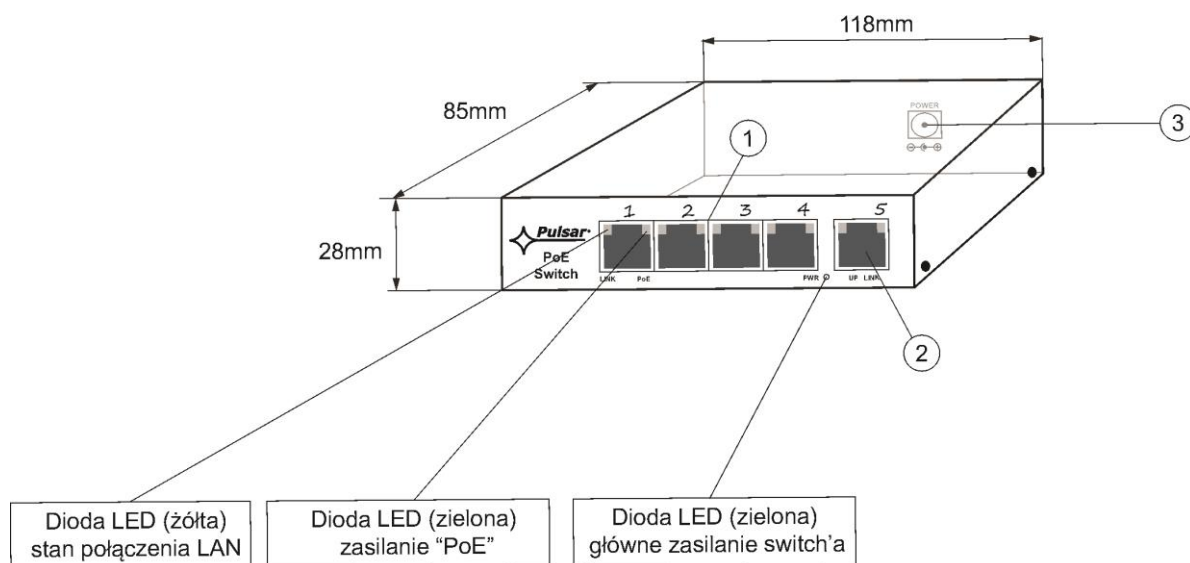
Rys. 3 Widok switch'a.
