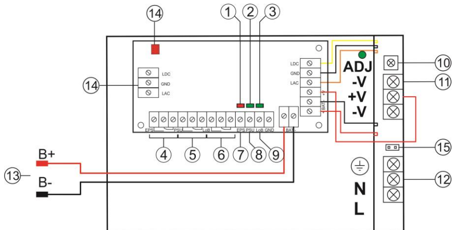
Obr. 2. Pohľad na zdroj.
