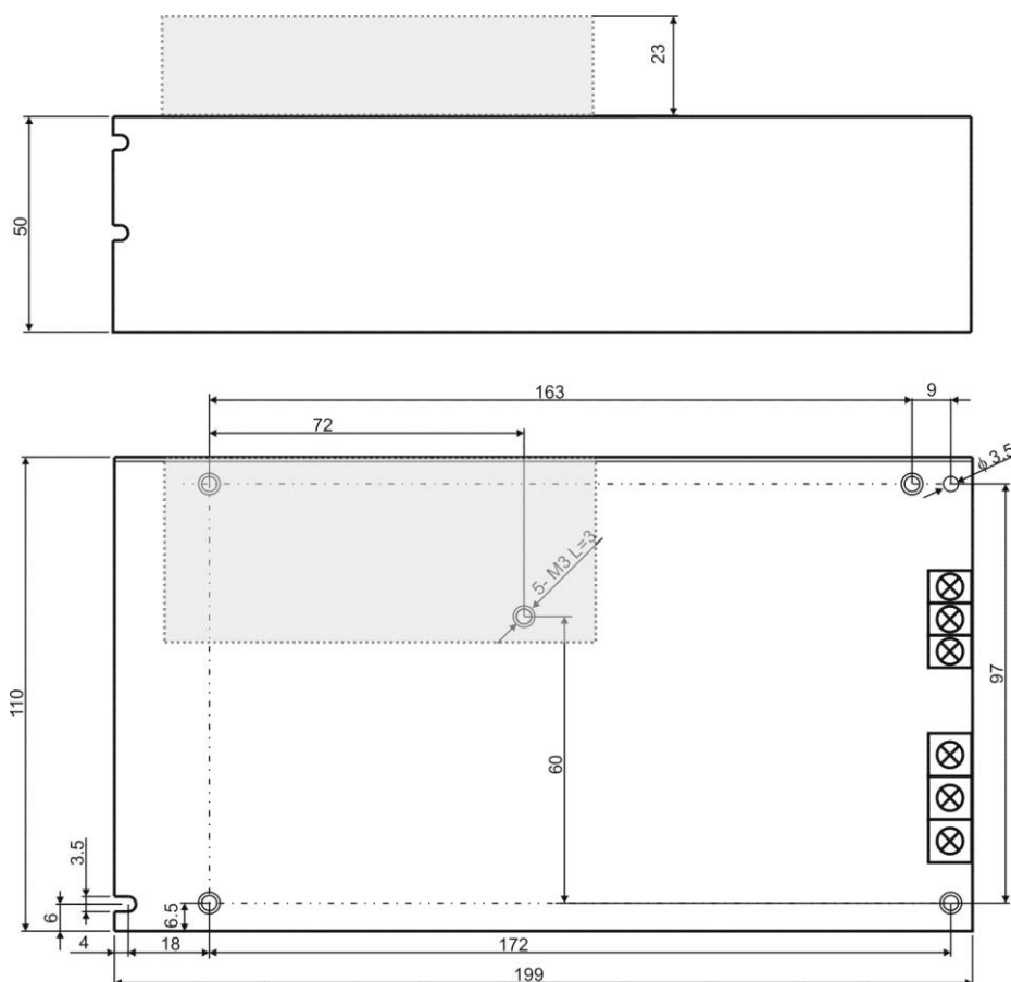
Obr. 3. Rozmery zdroja.
