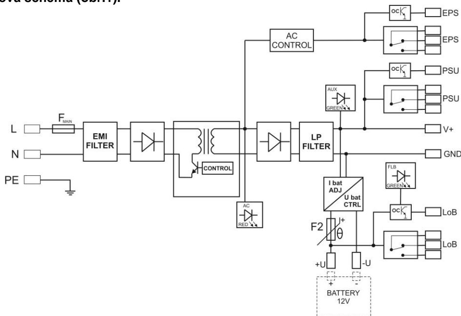
Obr.1. Bloková schéma zdroja.
